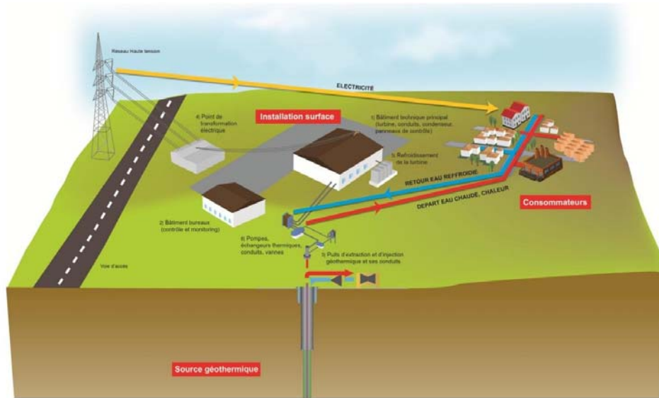
FONGEOSEC : circuit de valorisation énergétique (cliquez pour voir l'image agrandie)
